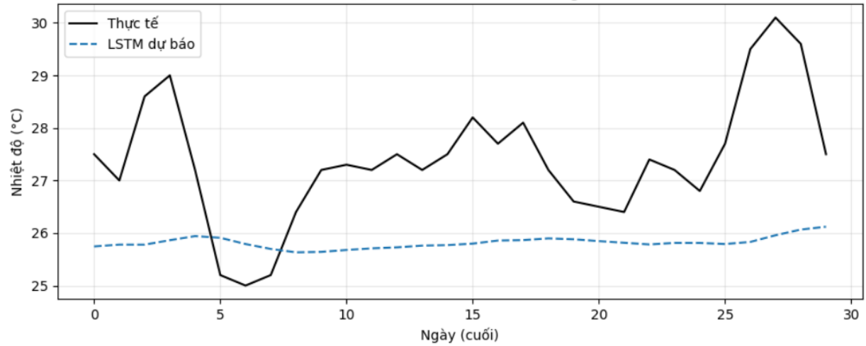
So sánh dự báo và thực tế - Đà Nẵng (LSTM)
